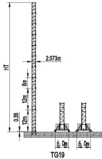
塔身组成 Tower configuration
